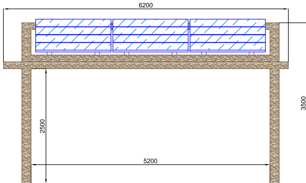
Vista frontale
