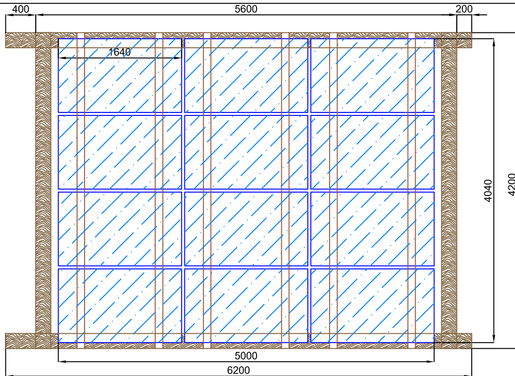
Vista dall'alto
