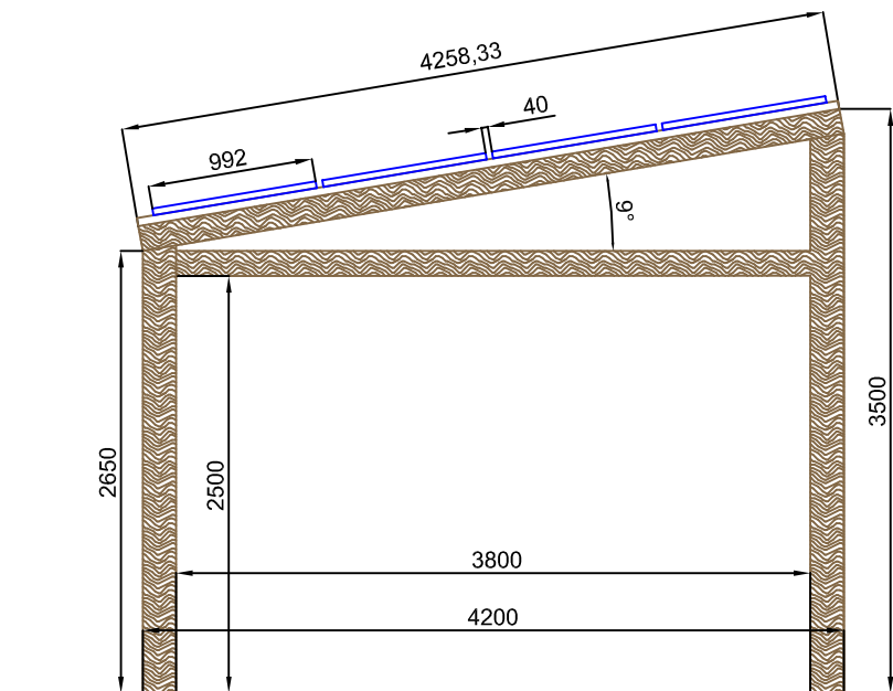
Vista laterale
